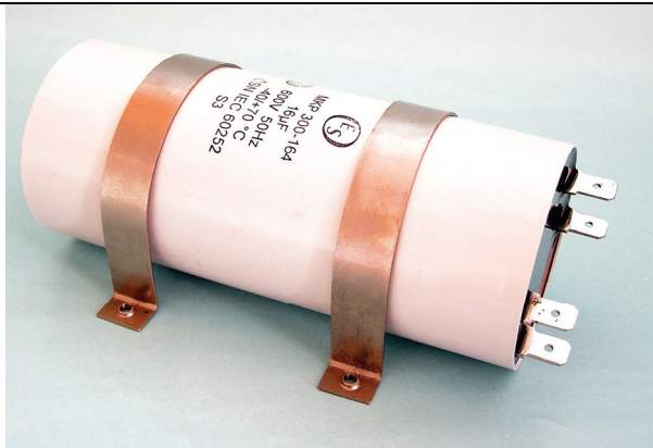
Tabulární kond. s příchýtkami
